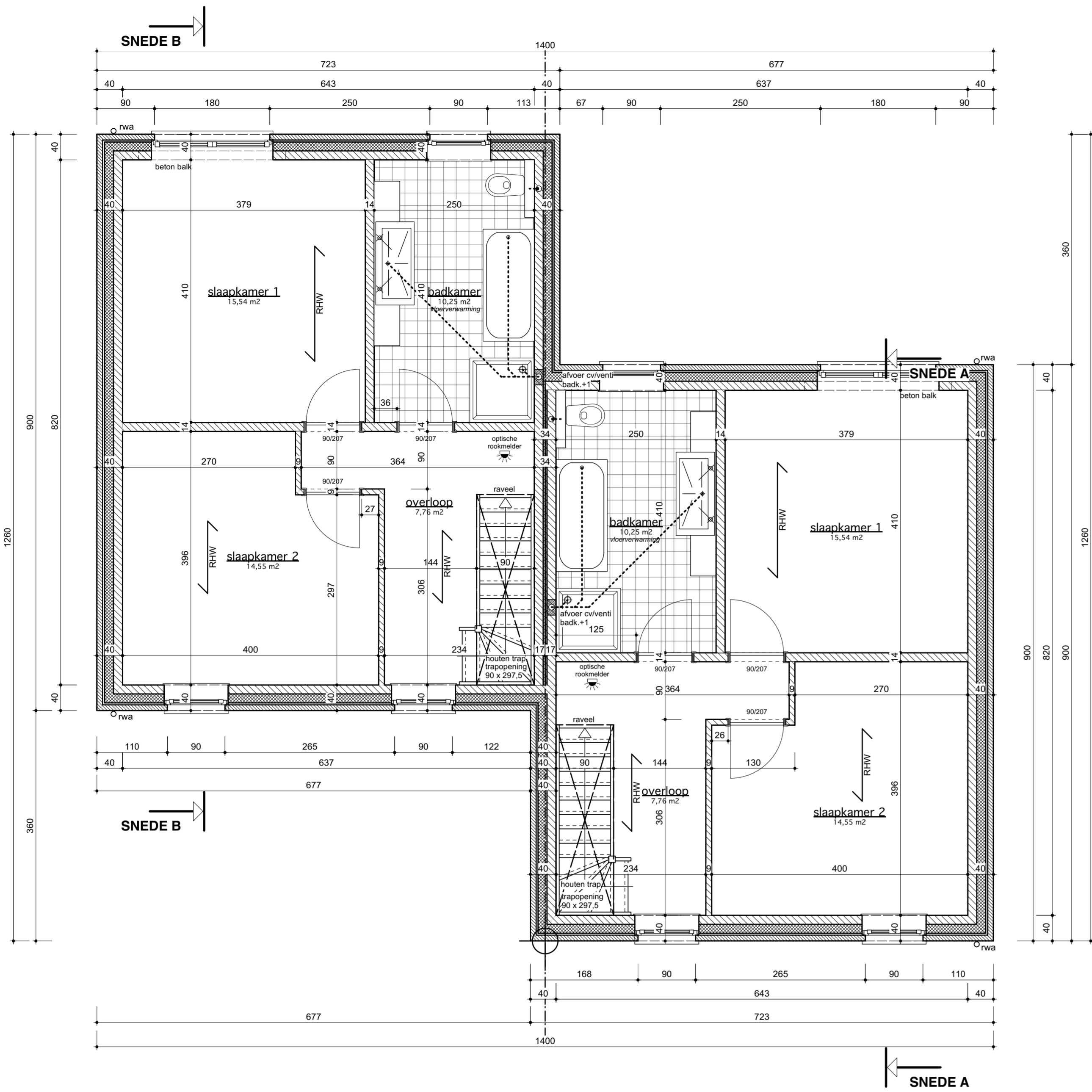
Verdiepingsplan Schaal: 1:50
