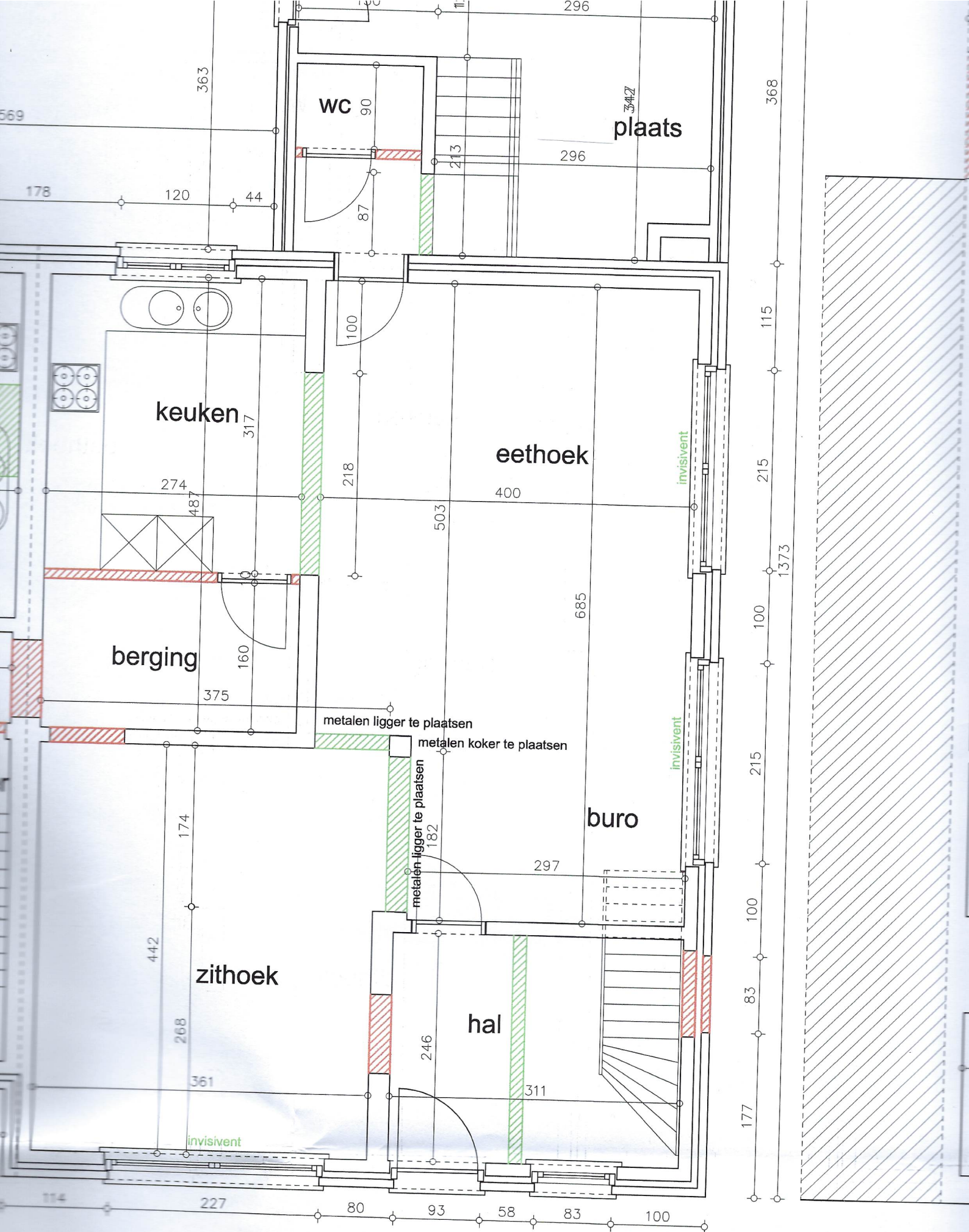
GRONDPLAN nieuwe toestand schaal 1/50
