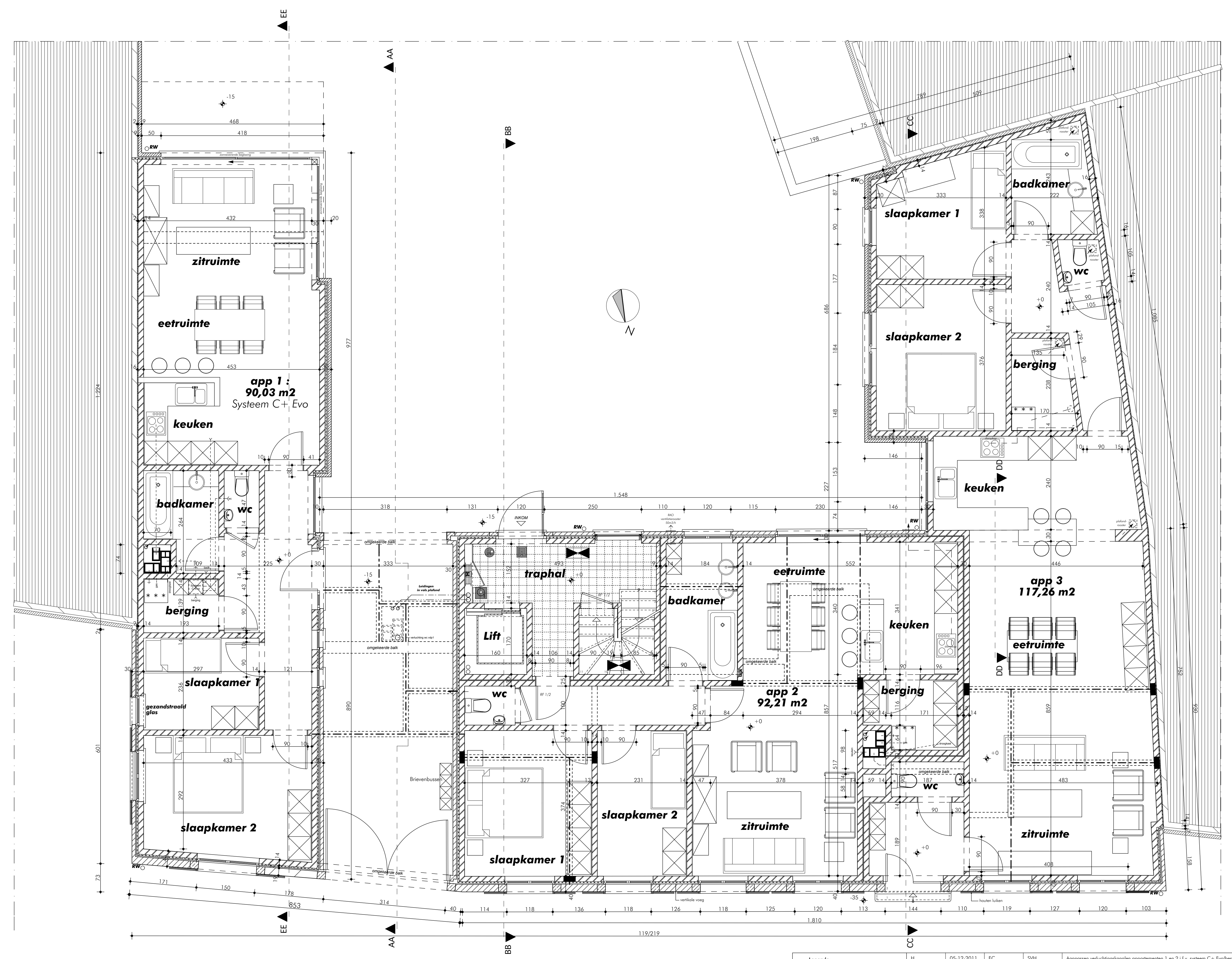
GRONDPLAN GELIJKVLOERS • nieuwe toestand
